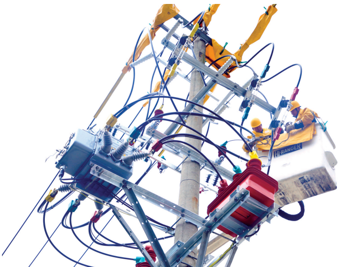
近日,南方电网贵州遵义桐梓供电局工作人员对10千伏东林线加装智能化自动开关投运开展带电作业。自动化开关的投运有利于维护人员及时了解、掌握配网运行状况,准确判定故障区段,缩短抢修处理时间,提高供电效率。
